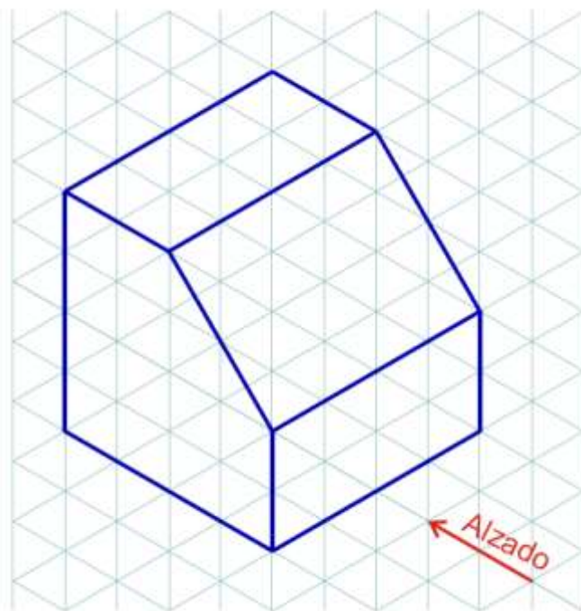
FIGURA 2. VISTAS PRINCIPALES
