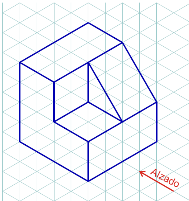
FIGURA 3. VISTAS PRINCIPALES
